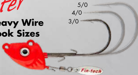
Hooks shown at actual size.
